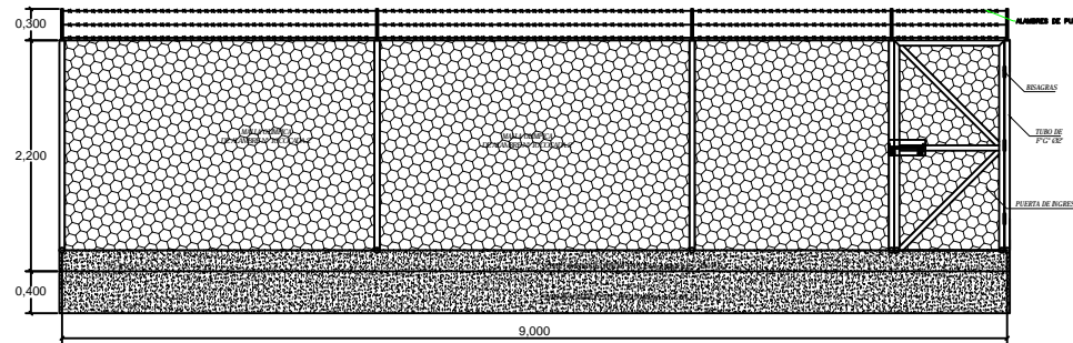
CERCO PERIMETRAL VISTA EN FRONTAL
