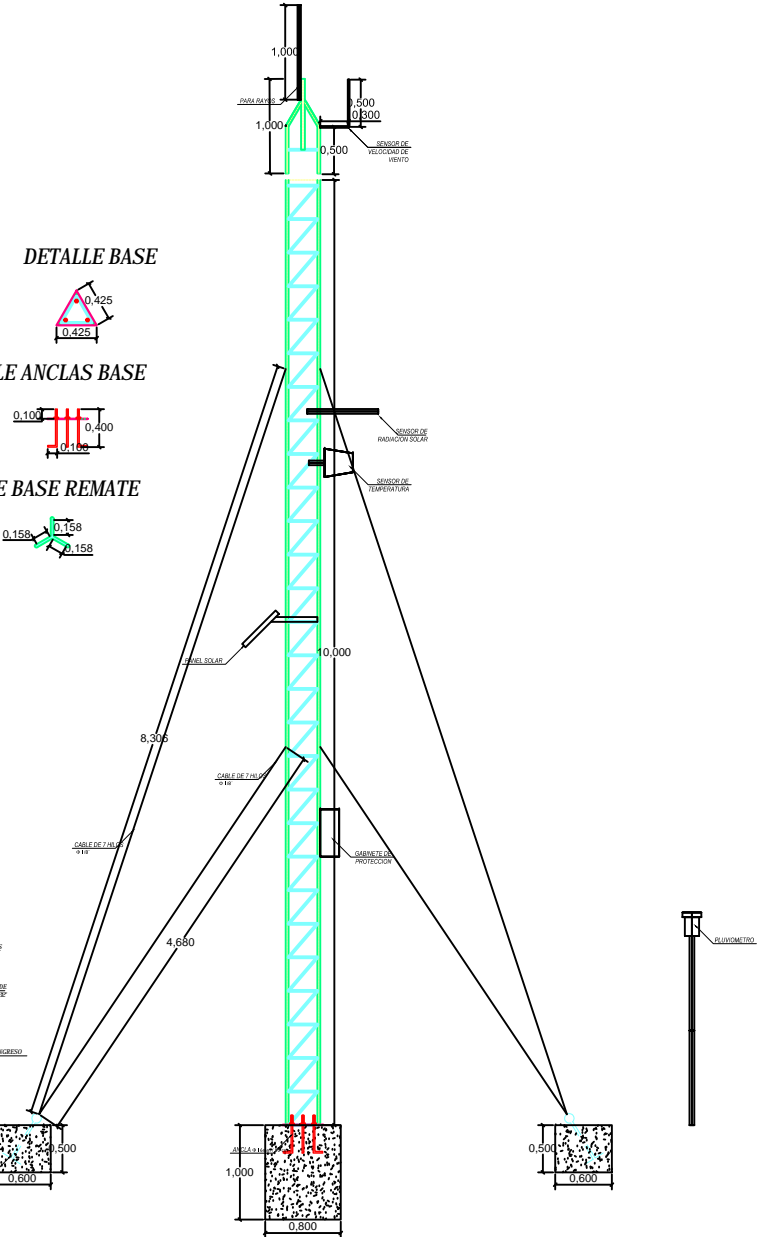
DETALLE TORRE VISTA FRONTAL
