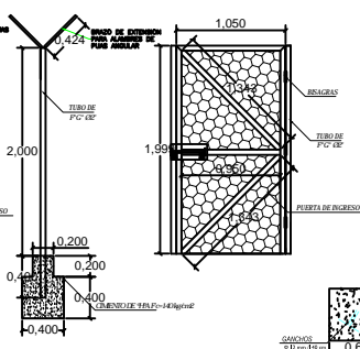
DETALLE PARANTE - PUERTA
