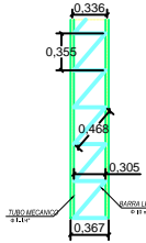
DETALLE CELOCIA TORRE
