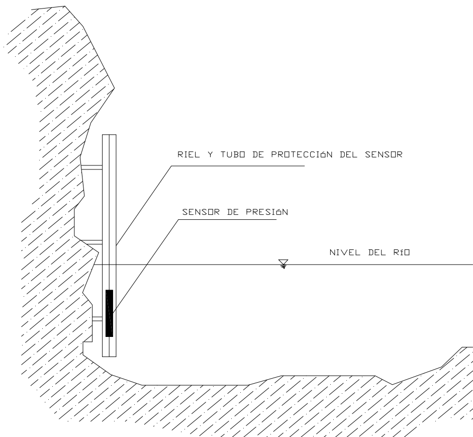
Figura 5. Esquema de instalación de estaciones de niveles con sensores hidrostáticos.
